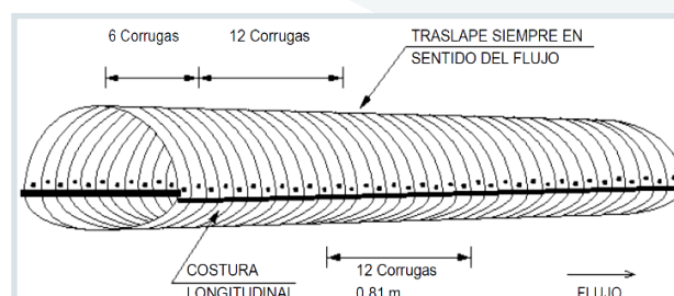
Sección ABOVEDADA
