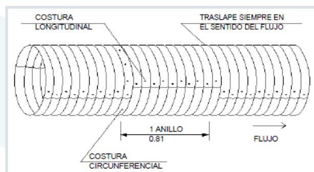
Sección CIRCULAR
