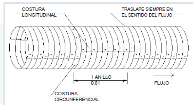
Sección CIRCULAR
